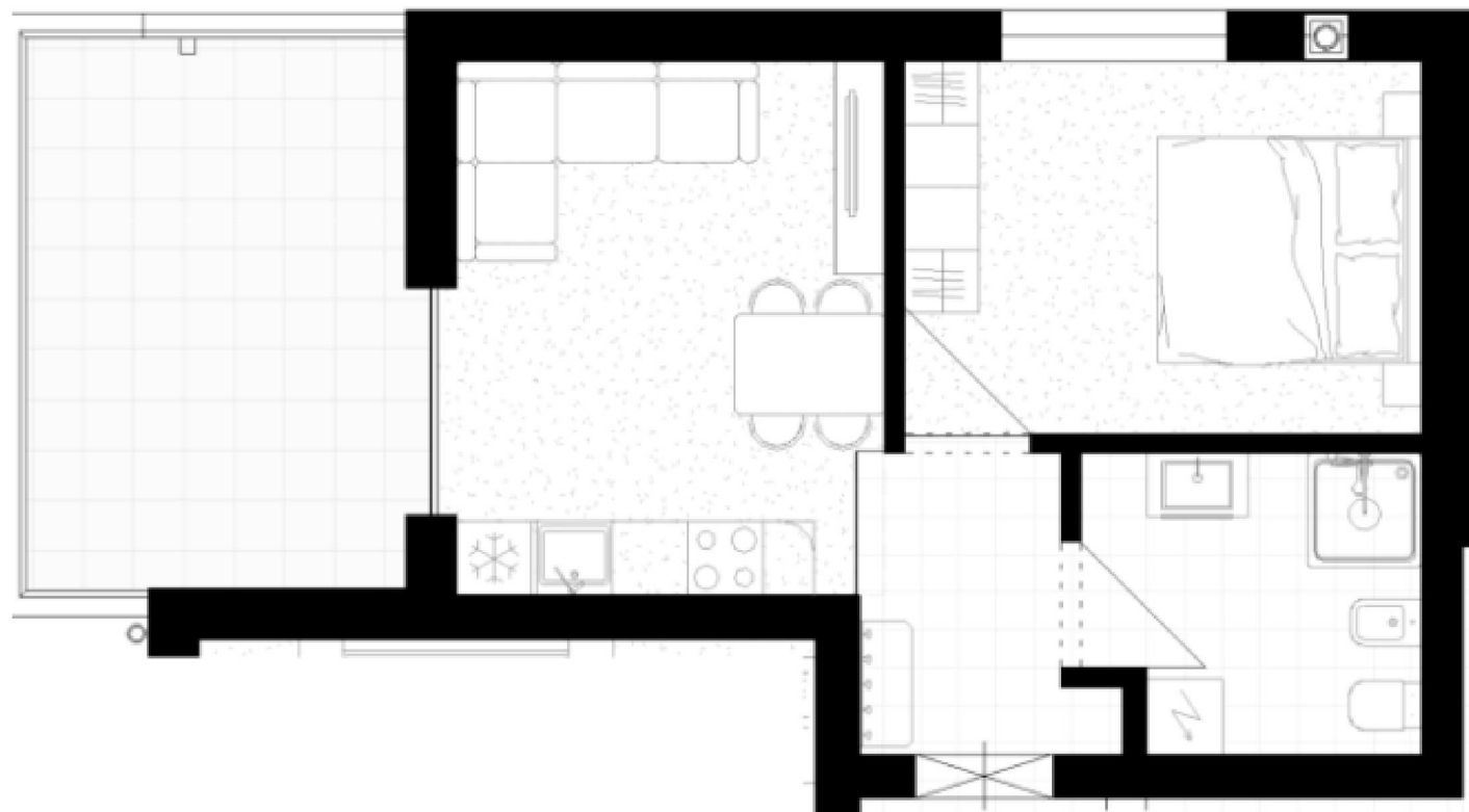
GRUNDRISS WOHNUNG 8
